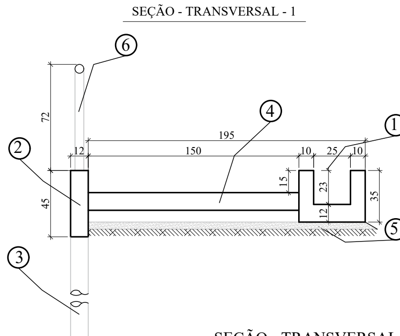
SEÇÃO - TRANSVERSAL
